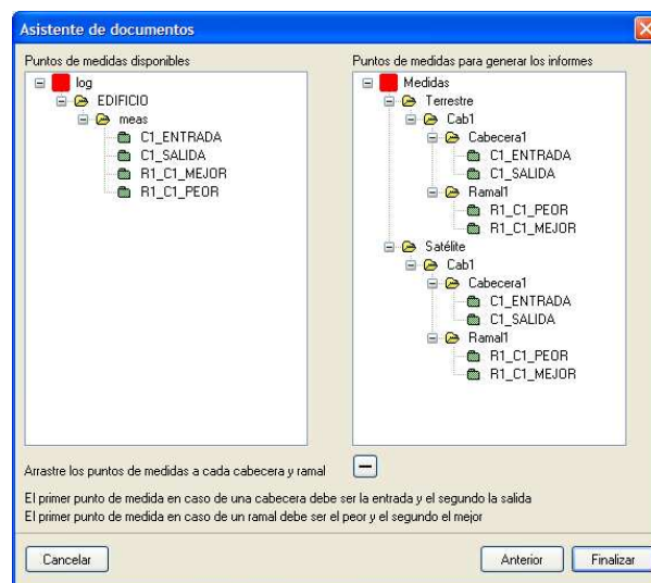
Ilustración 103: Colocando puntos de medidas de una instalación ICT
