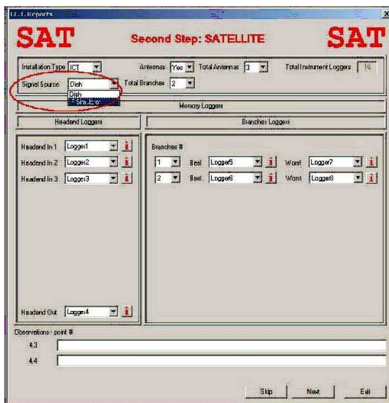
Ilustración 109 informe relativo a la distribución de señales Satélite o con Simulador de portadoras
